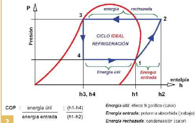
CICLO REFRIGERACIÓN IDEAL DIAGRAMA PRESIÓN – ENTALPÍA
